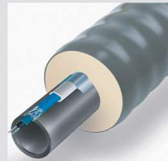
ТВЭЛ-ЭКОПЭКС-ХВС с кабель-каналом
